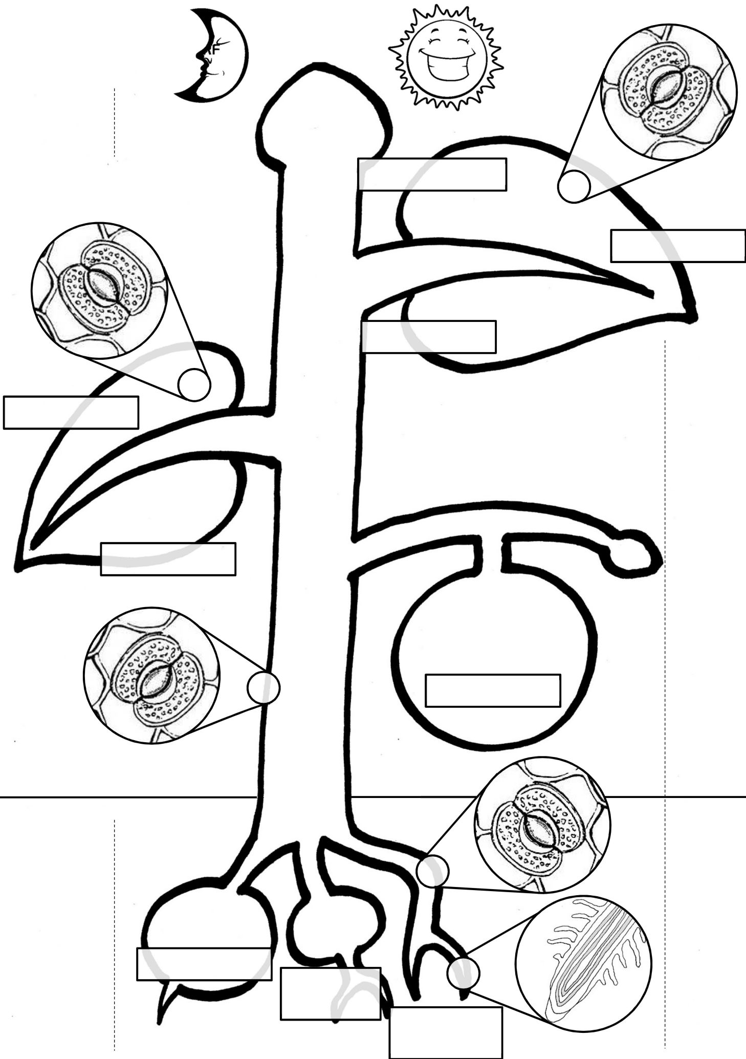
Schéma bilan de la nutrition et de la fabrication d'énergie chez les végétaux
